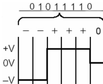
Rys.11 Przykładowe kodowanie systemem 8B/6T-[2]
