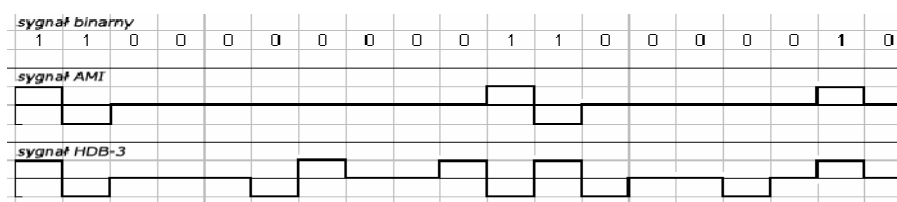
Rys.15 przykładowe kodowanie sygnału binarnego do kodu AMI oraz HDB-3. –[3]
