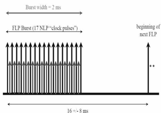
Rys. 18. Sposób kodowania słów FLP –[8]
