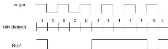
Rys. 4 Sposób kodowania NRZ - [4]
