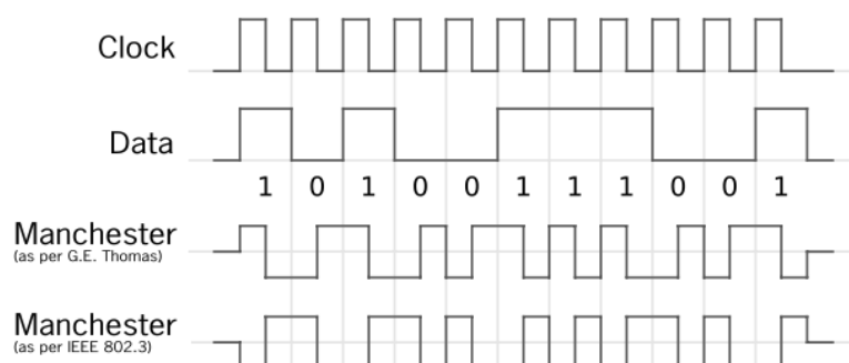
Rys.1. Modulacja sygnału cyfrowego za pomocą kodu Manchester - [ 2 ]
