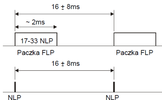
Rys.17. Długość trwania słów FLP i NLP –[8]
