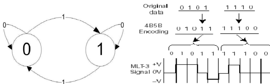
Rys. 8 Zasada działania kodu MLT-3-[2] Rys. 9 Przykładowy ciąg danych zakodowanych w MLT-3-[ 2 ]
