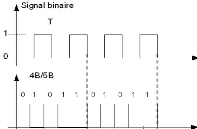
Rys. 7 Sposób kodowania kodem 4B/5B
