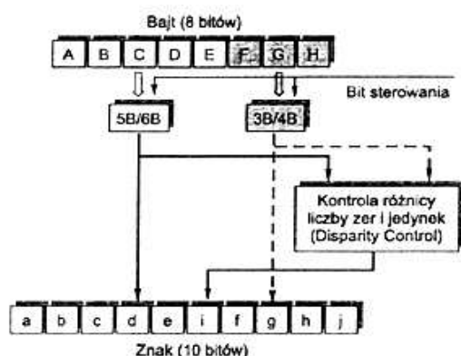
Rys. 12 Schemat kodowania 8B/10B-[2]
