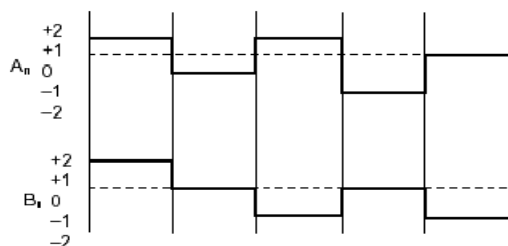
Rys. 14 Przykładowy kod PAM-5-[2]
